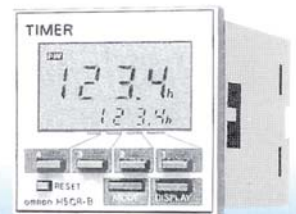
AUTO-STARTER (EXCEPT 242HS-A)
